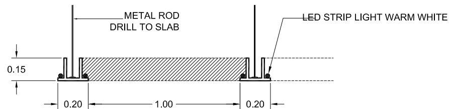
A17 3 SCALE 1:100M SECTION A-A
