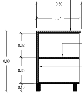
A-15 04 TYP. SECTION A-A SCALE 1:50 M
