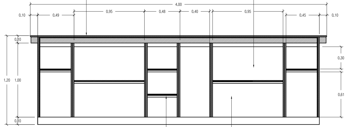
A-16 04 SECTION A-A SCALE 1:50 M
